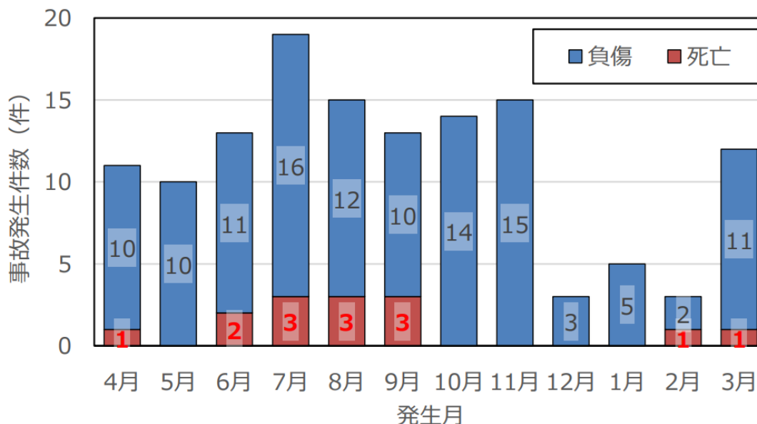
[図4] 発生月別・被害別の感電死傷事故件数 (2019～2021年度)
